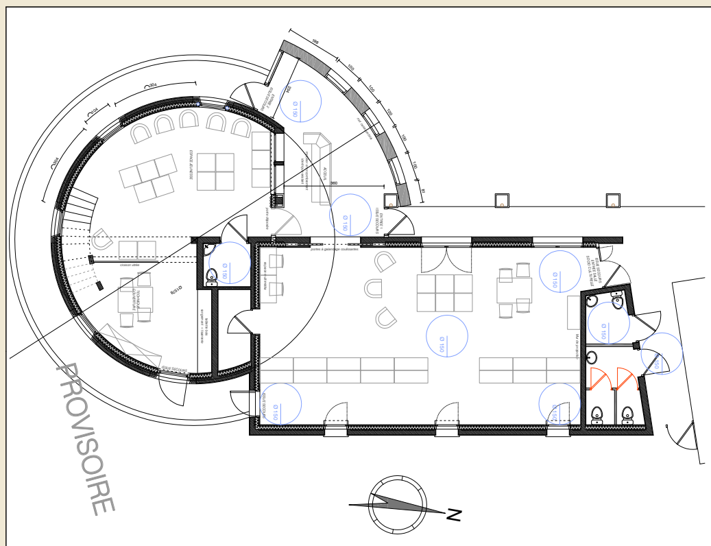
▲ Esquisse de projet de l'extension/aménagement de la Bibliothèque – Plan de niveaux Rez-de-chaussée
